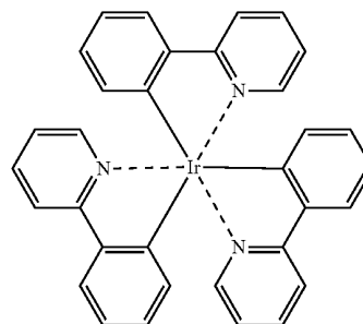
Ir(ppy) 3
