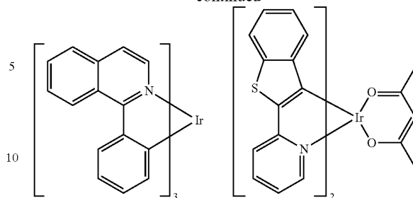
Ir(piq) 3
