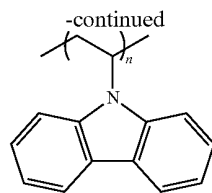
PVK
