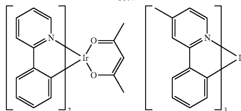
Ir(ppy) 2 (acac)
