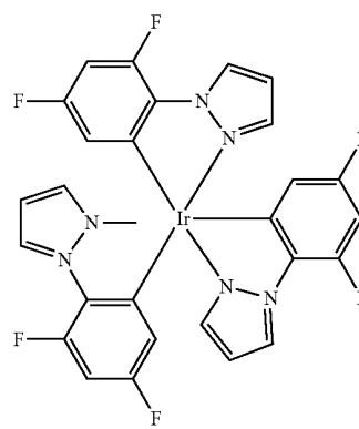
Ir(dfppz) 3
